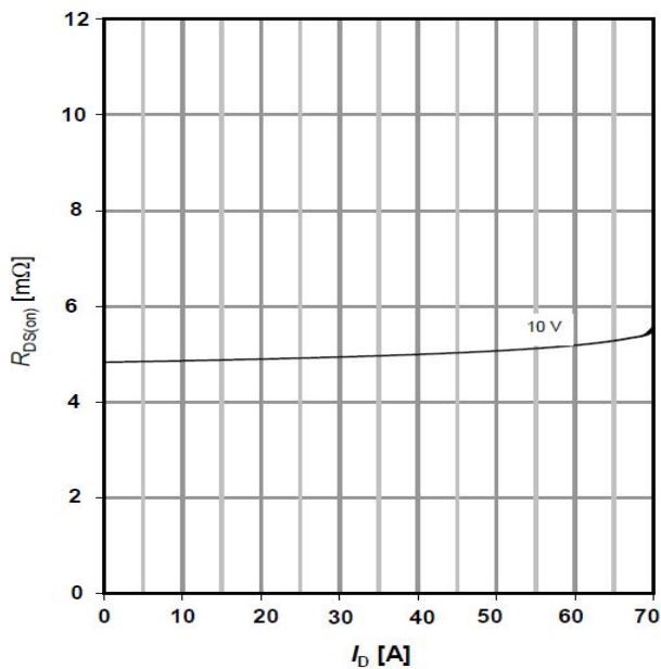
RDS(on) -- ID
